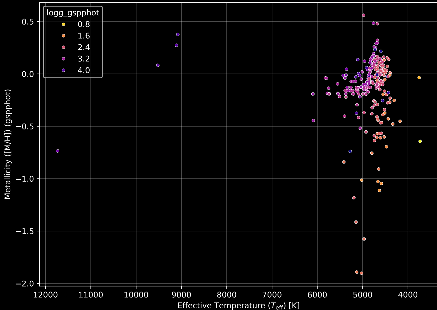
APOGEE DR17 Field: [340-10] Stellar Population Parameters (n= 244)
